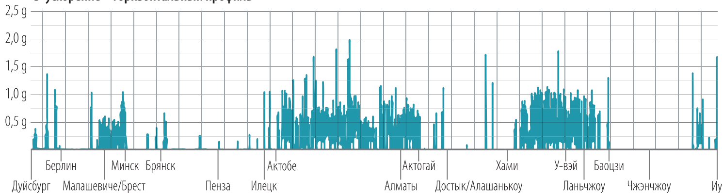
G-ускорение – горизонтальный профиль
